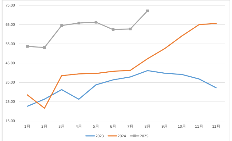
铁锂动力电池产量 72 月变动 9.4 年变动 30.9
