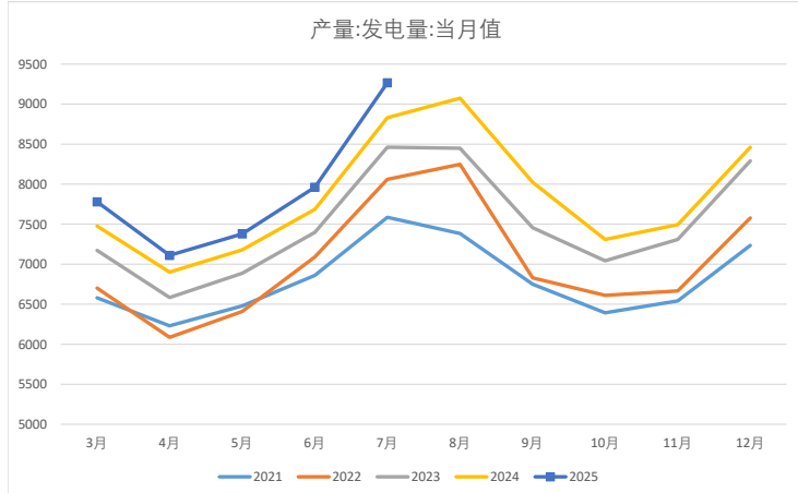
发电量 9267 月变动 1304 年累计同比 1.3% 年变动 436
