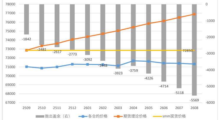
基于同一时间维度的期货价格考量 (2025年9月11日)
